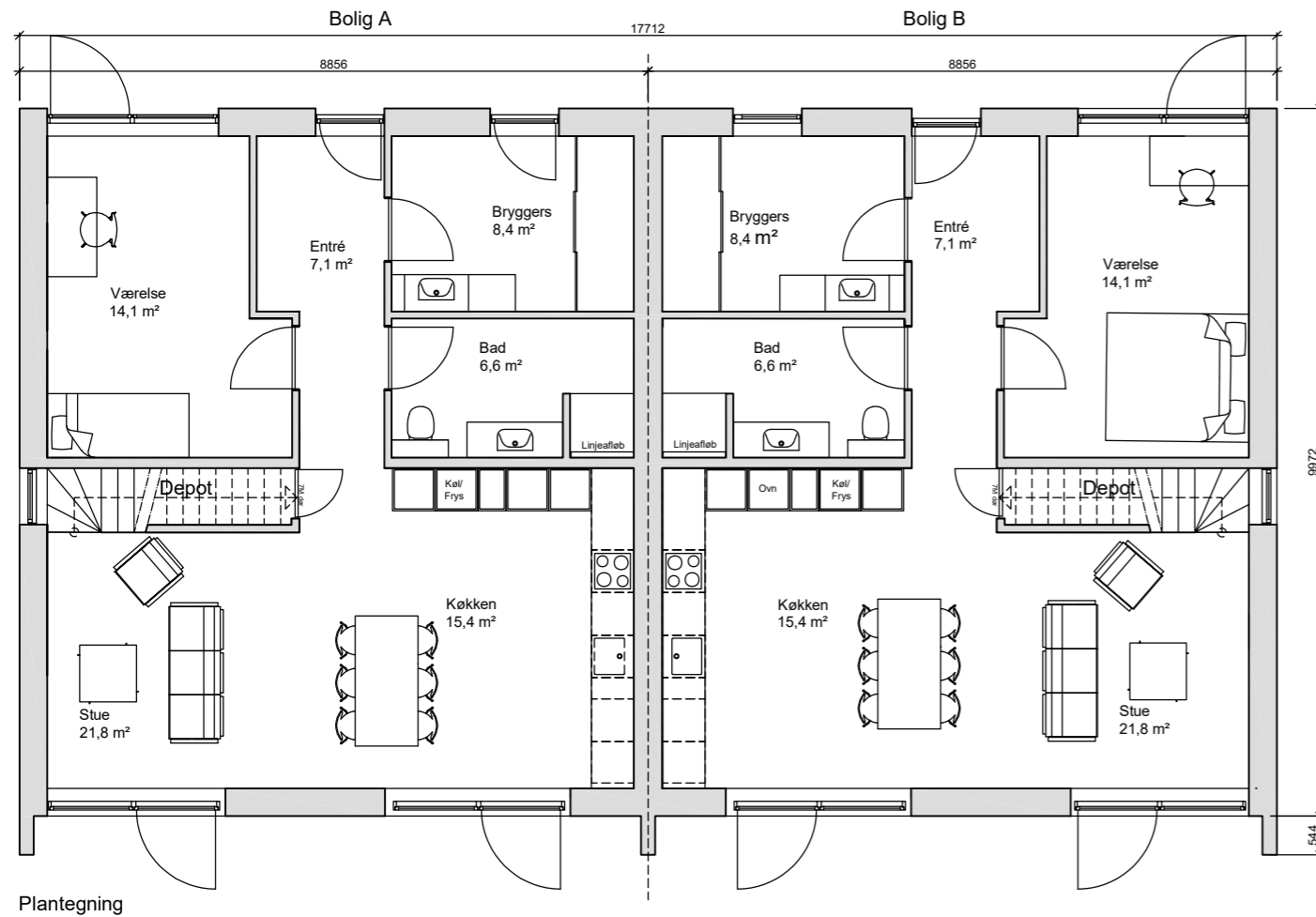
Plantegning
